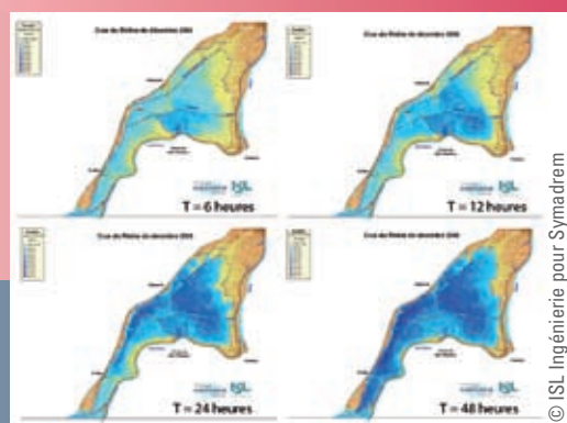
Résultat de la modélisation cinétique de la crue du Rhône de 2003
