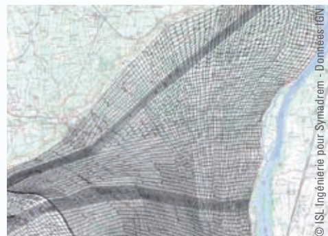
Mailles du modèle hydraulique
